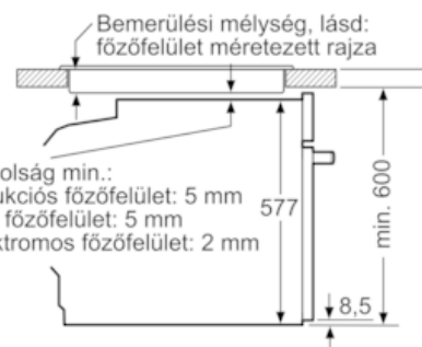
Méretetek mm-ben
