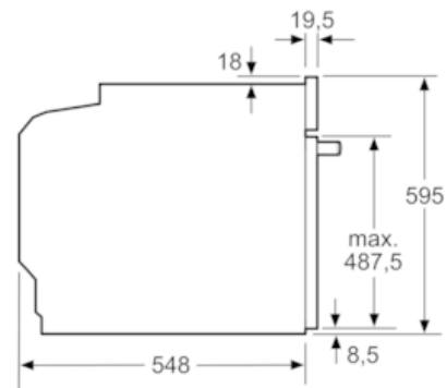
Méretetek mm-ben
